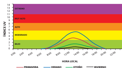
RADIACIÓN ULTRAVIOLETA COMPORTAMIENTO DIARIO ESTACIONAL ESTACIÓN PUNTA ARENAS
