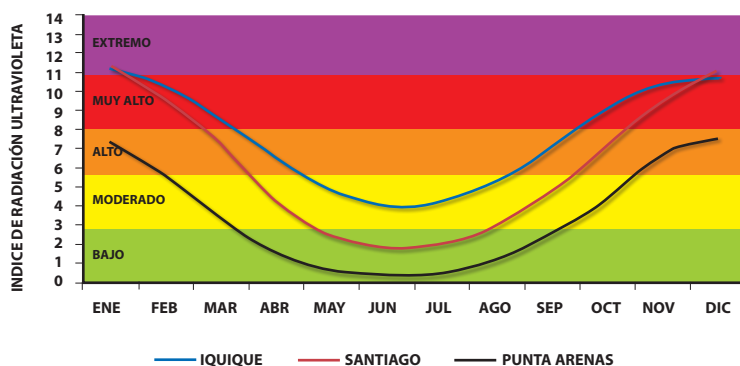
COMPORTAMIENTO ANUAL IUV-B PERIODO 2001 - 2010
