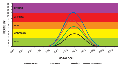
RADIACIÓN ULTRAVIOLETA COMPORTAMIENTO DIARIO ESTACIONAL ESTACIÓN IQUIQUE
