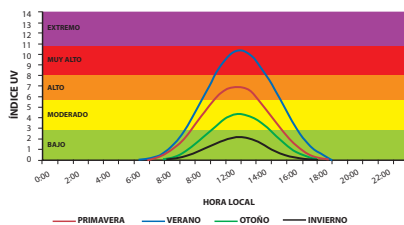
RADIACIÓN ULTRAVIOLETA COMPORTAMIENTO DIARIO ESTACIONAL ESTACIÓN SANTIAGO
